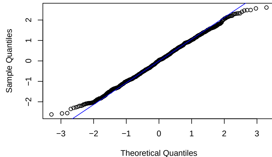
QQ normal do EAP padronizado
