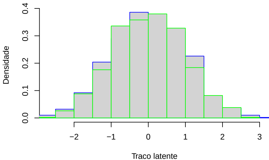
Verdadeiro (azul) e EAP (verde)
